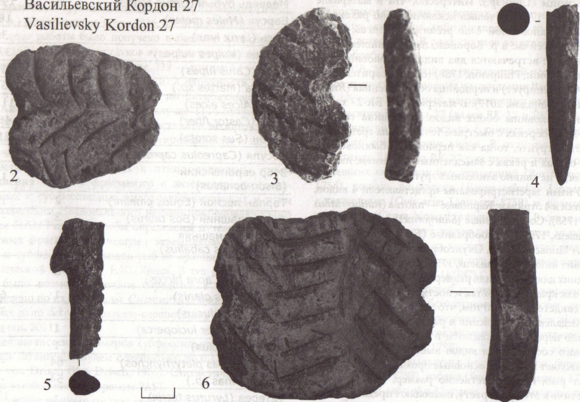
Рис. 1. 1 — местонахождение памятника археологии Васильевский Кordon 27 на карте Черноземья; 2-3, 6 — керамические грузики, 4-5 — обломки костяных гарпунов.
